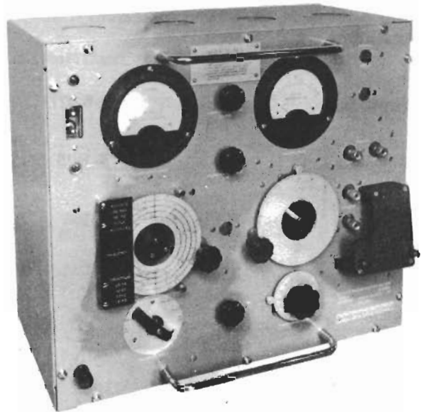
A.P. 100320 Q-METER
